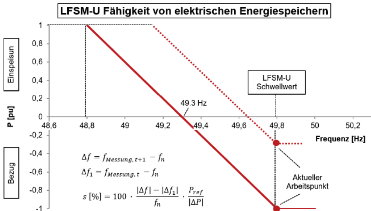
Abbildung 3: Fähigkeit von elektrischen Energiespeichern zur frequenzabhängigen Anpassung der Wirkleistung im LFSM-U-Modus (Darstellung für P_{ref} = P_{max,E} und s = 1 \% )
