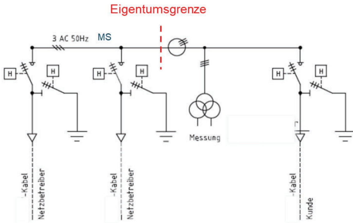
Abbildung 11: Ausführungsbeispiel mit Übergabestation zum kundeneigenen MS-Netz
