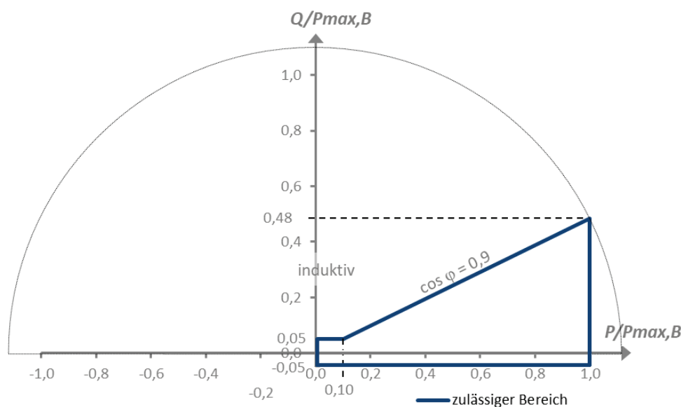
Abbildung 7: Zulässiger Blindleistungsbereich für Kundenanlagen ( Q ist die Blindleistung der Kundenanlage in var, P ist die Wirkleistung der Kundenanlage in W, P_{max,B} ist die maximale Bezugskapazität der Kundenanlage in W und \cos \varphi ist der Verschiebungsfaktor)
