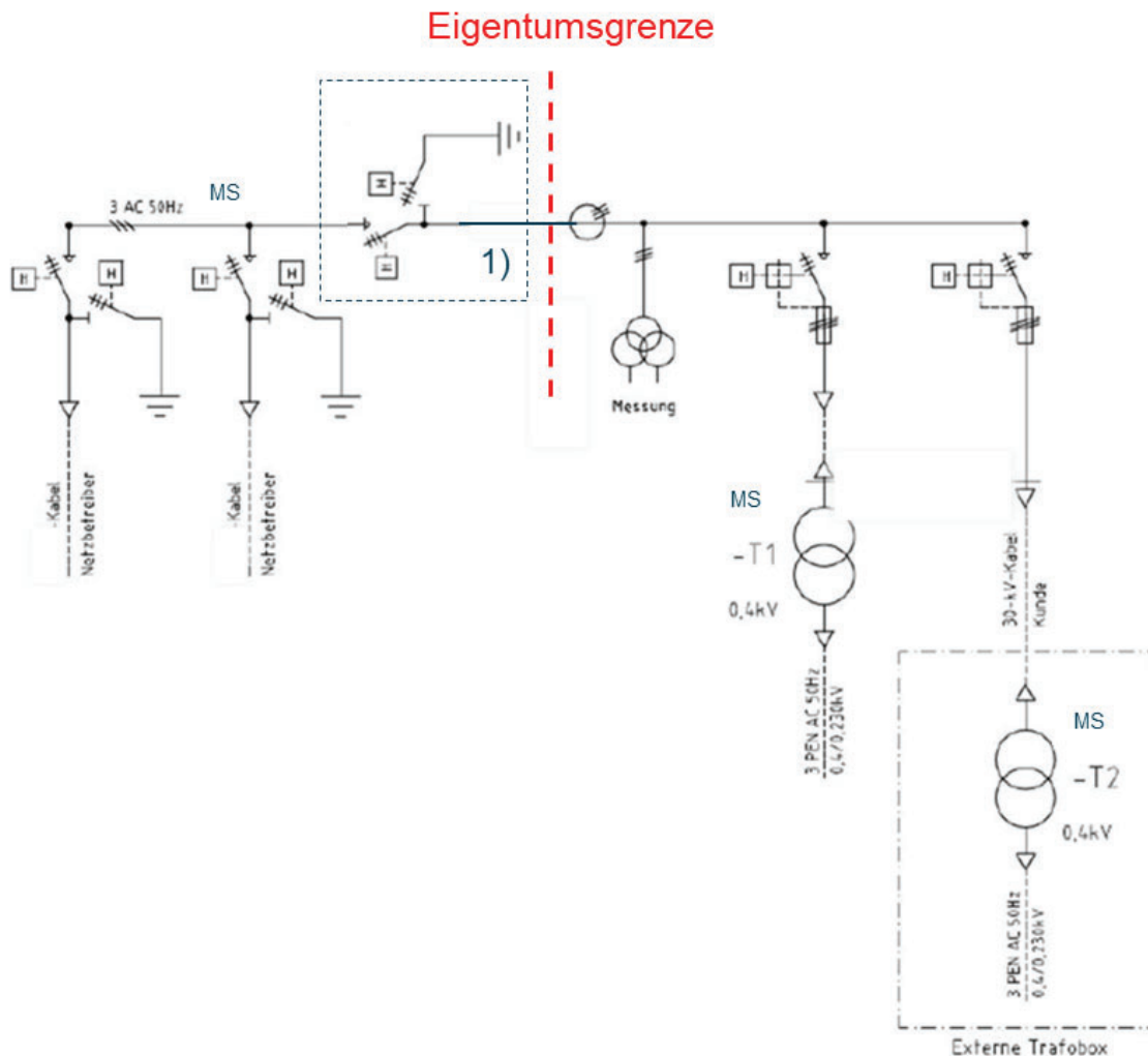
Abbildung 10: Ausführungsbeispiel mit mehreren Trafoabgängen
