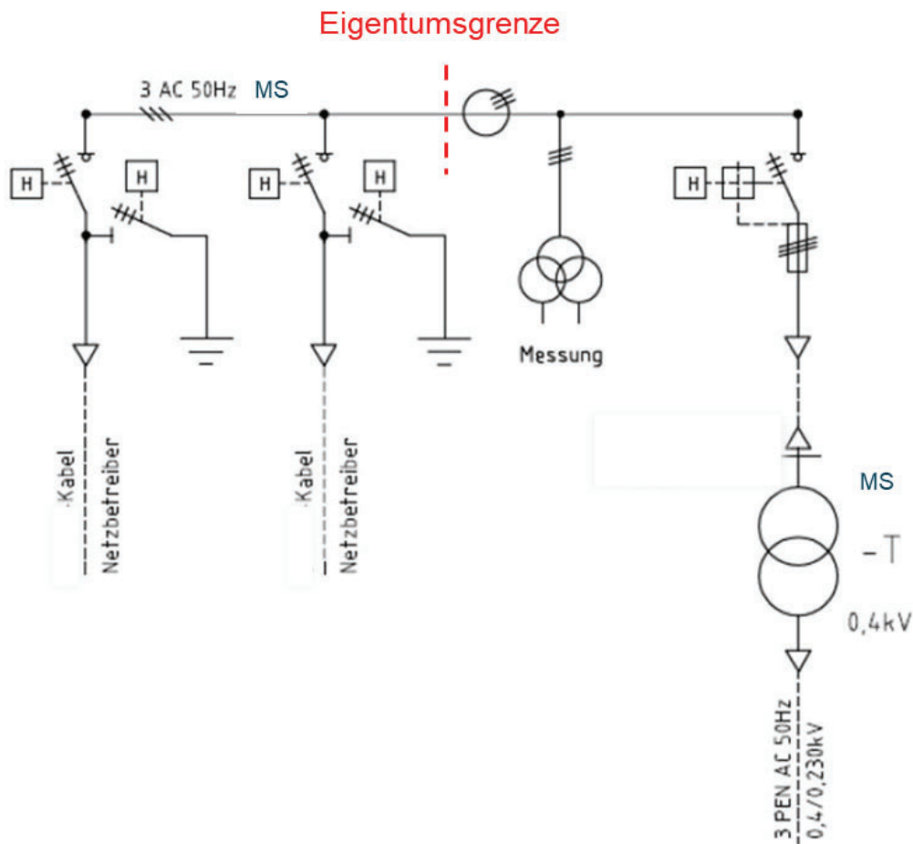
Abbildung 9: Ausführungsbeispiel mit einem Trafo
