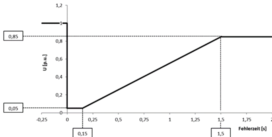
Abbildung 6: FRT-Profil mit Netzanschlusspunkt auf MS-Ebene
