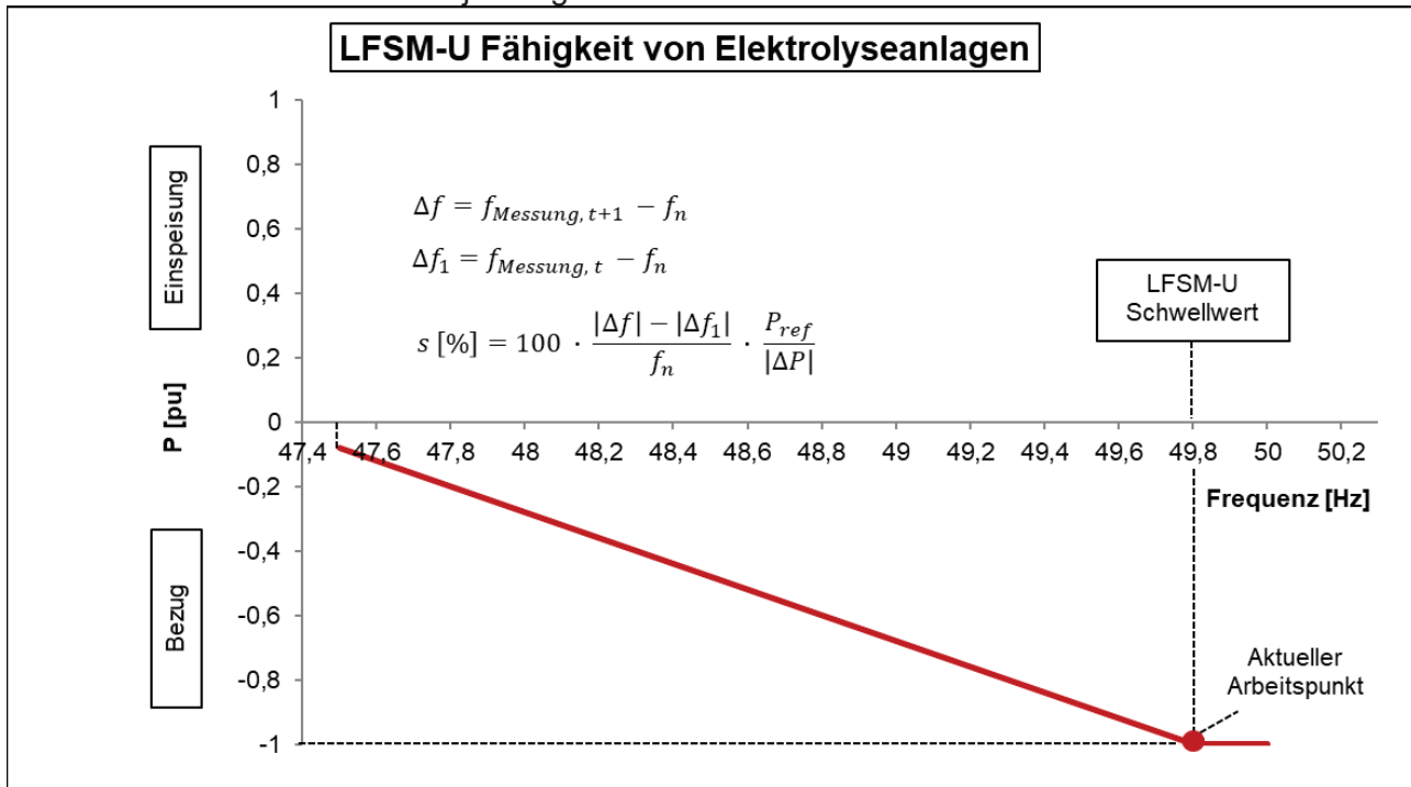
Abbildung 5: Fähigkeit von Elektrolyseanlagen zur frequenzabhängigen Anpassung der Wirkleistung im LFSM-U-Modus (Darstellung für P_{\text{ref}} = P_{\text{nom}} und s = 5 \text{ \%} )
