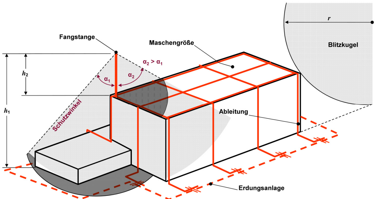
Bild 2 – Verfahren für die Auslegung von Fangeinrichtungen und Ableitungen
