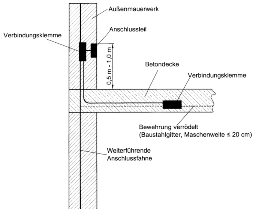
Bild A.2 – Beispiel für ein vertikales Anschlussstück im Obergeschoss für EMV-Maßnahmen
